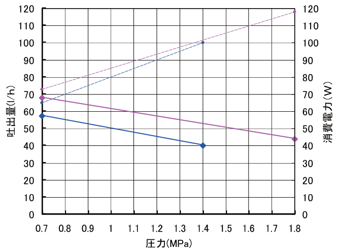
●GFS-VEA 消費電力・吐出量
