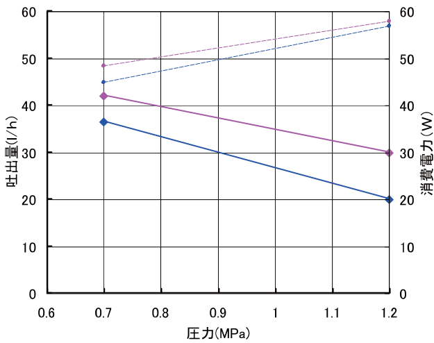
●GFS-VA 消費電力・吐出量
